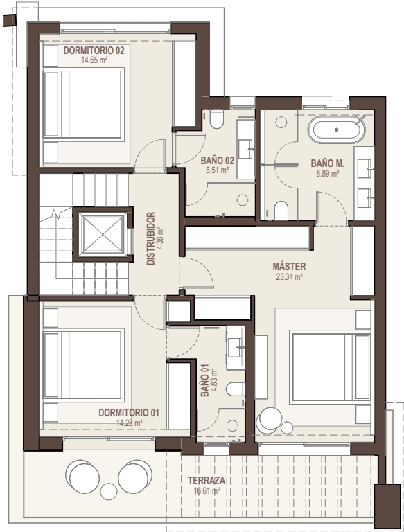
PLANTA ALTA 1 : 100
