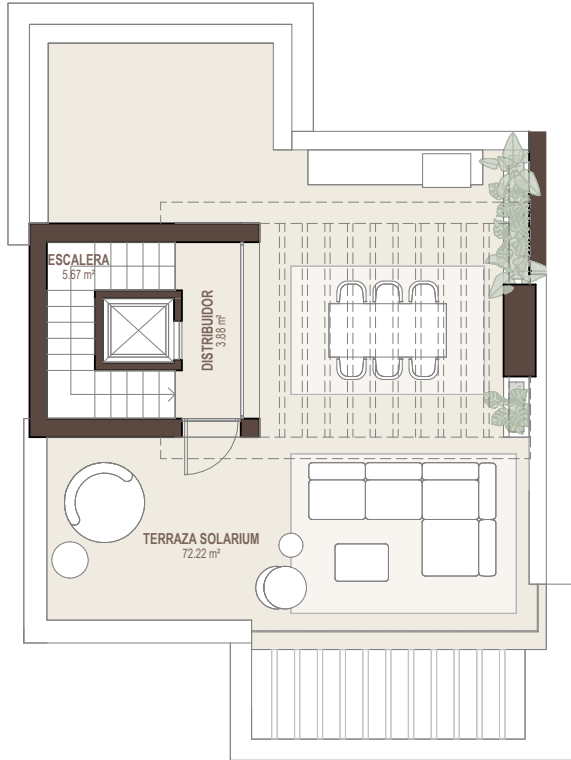
PLANTA SOLARIUM 1 : 100
