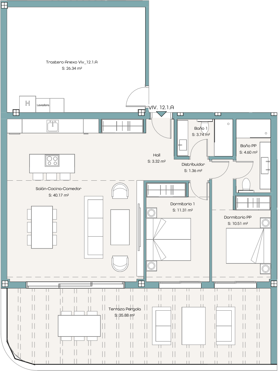
PLANTA PRIMERA
