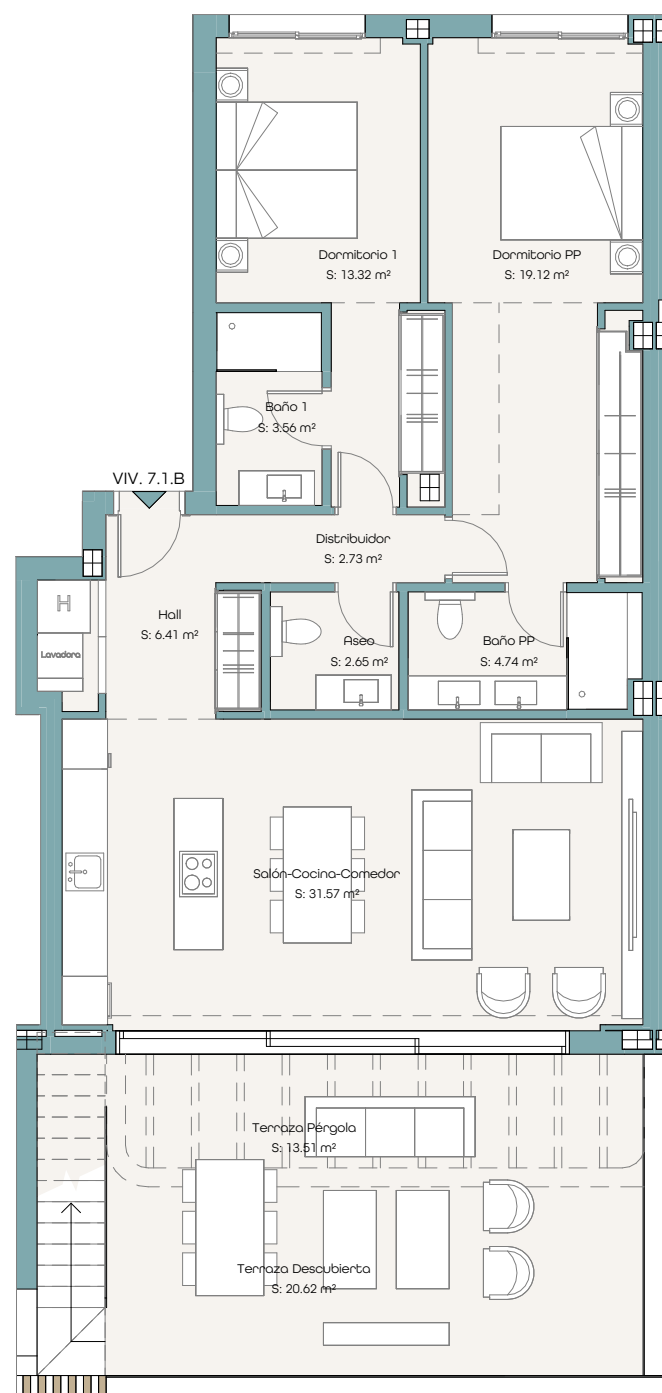
PLANTA PRIMERA
