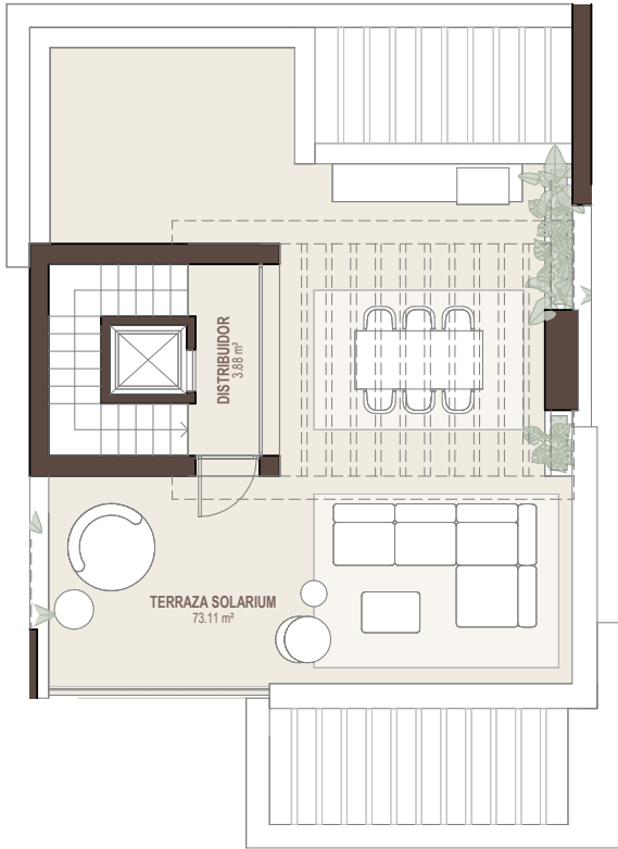
PLANTA SOLARIUM 1 : 100
