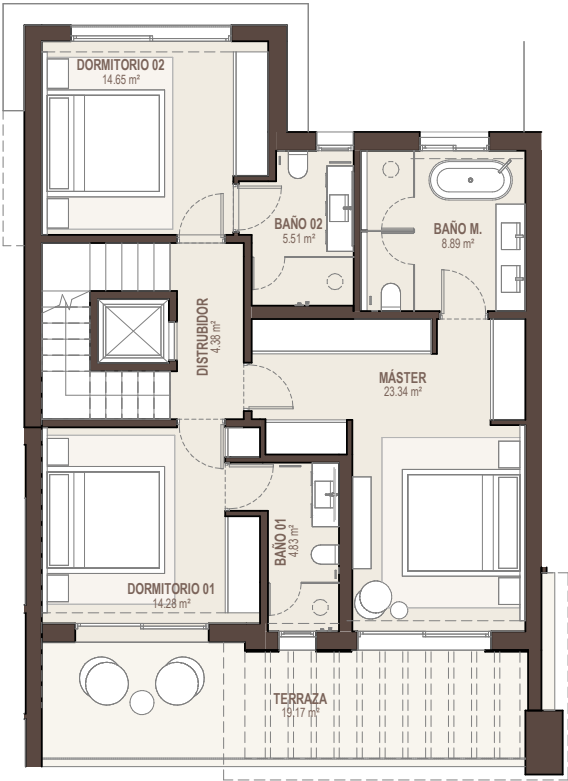
PLANTA ALTA 1 : 100
