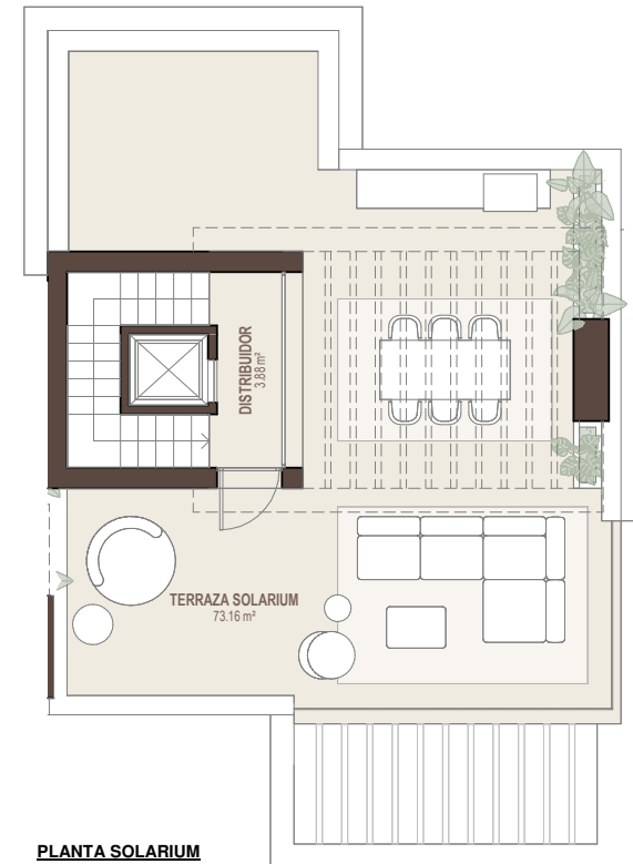
PLANTA SOLARIUM 1 : 100
