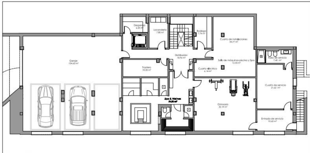
Planta sótano (Nivel 59,35)
