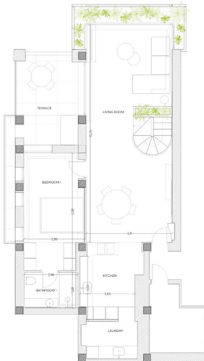
PLANTA BAJA
