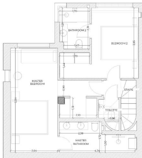
PLANTA -1
