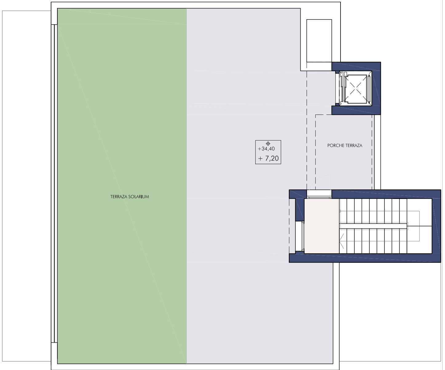
PLANTA TERRAZA
