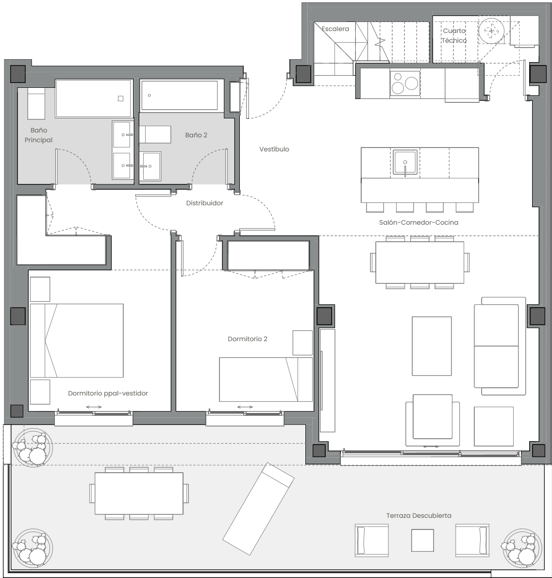
PLANTA ACCESO_P04
