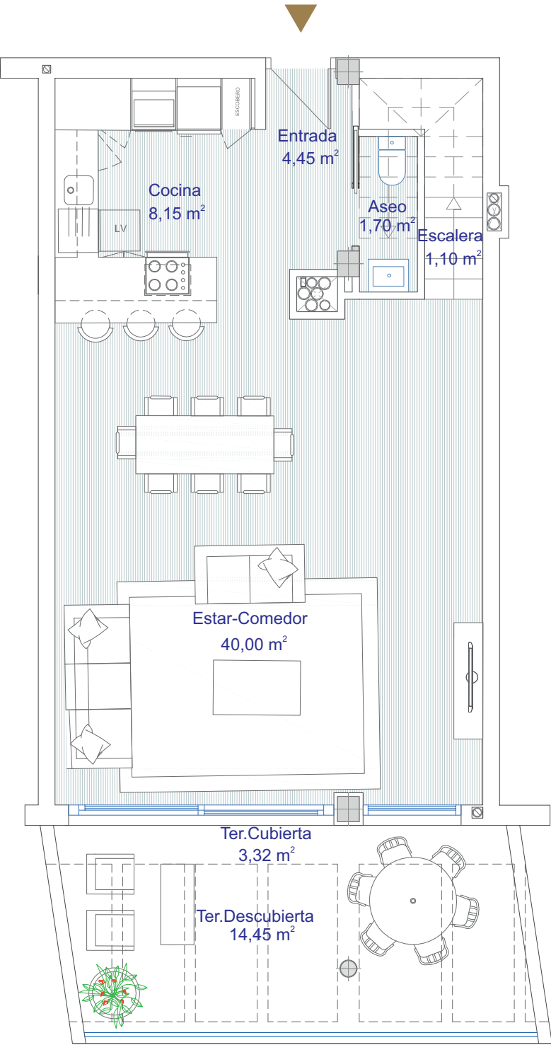
NIVEL 3
