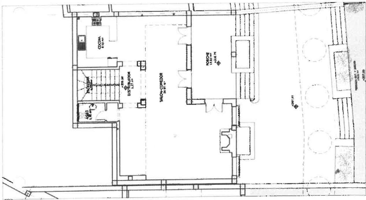
PLANTA 2 COTA +208.00 m
