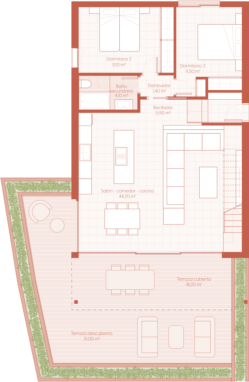
PLANTA BAJA
