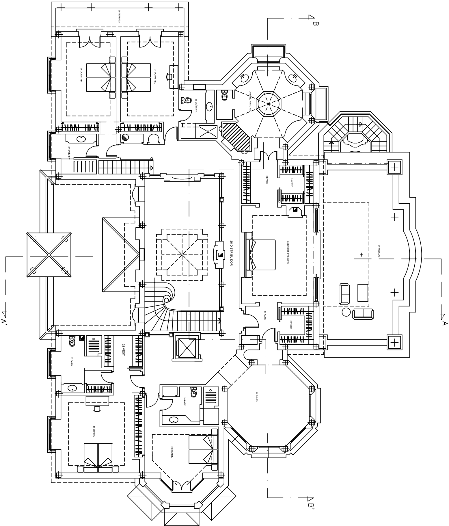
PLANTA ALTA
