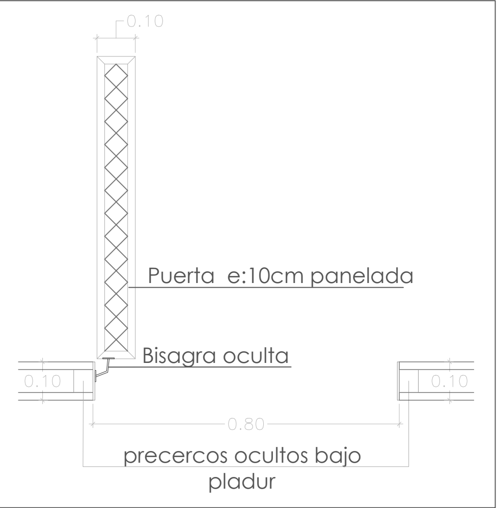
DETALLE PUERTA E:1/10
