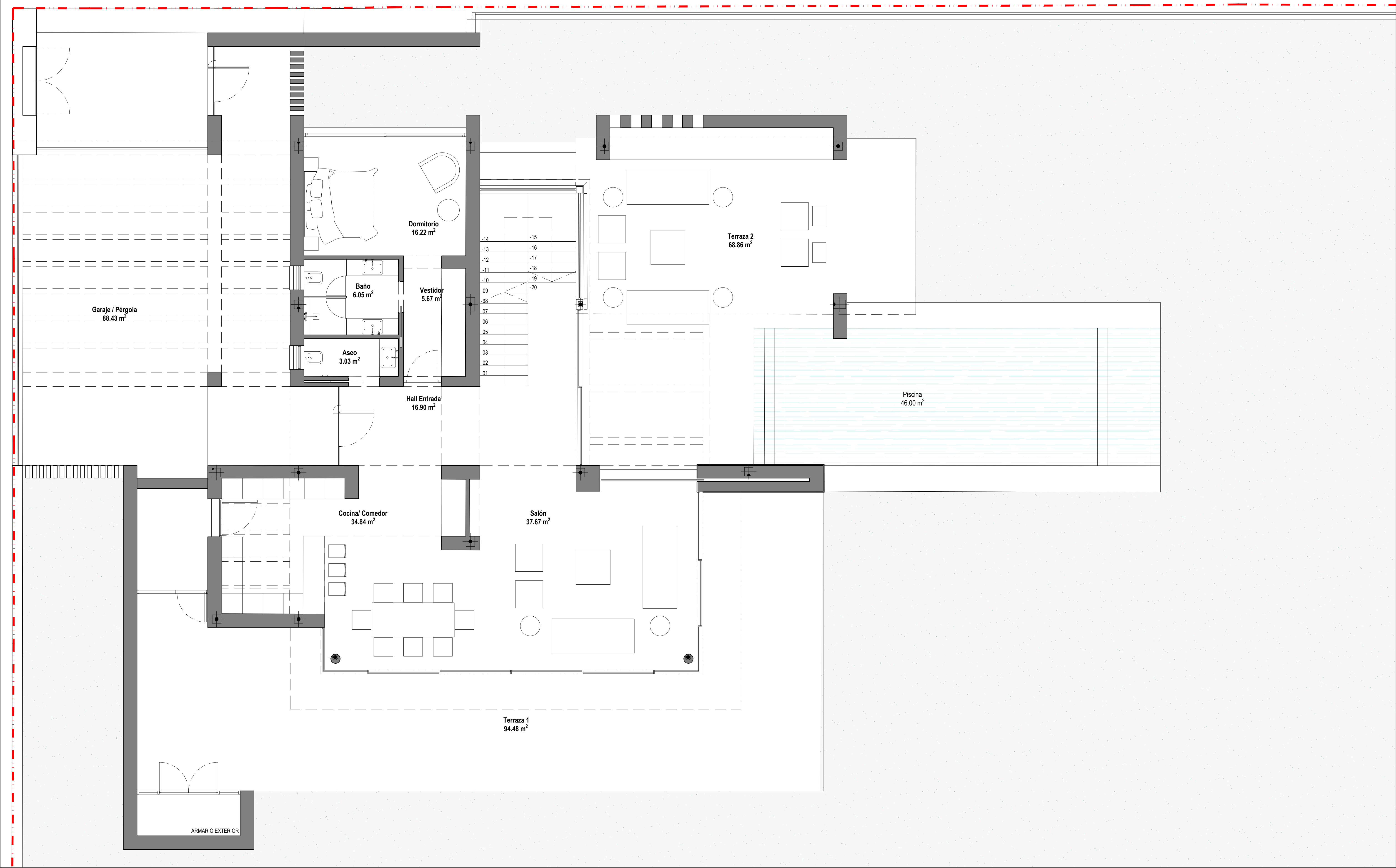
PLANTA BAJA_E:1.50
