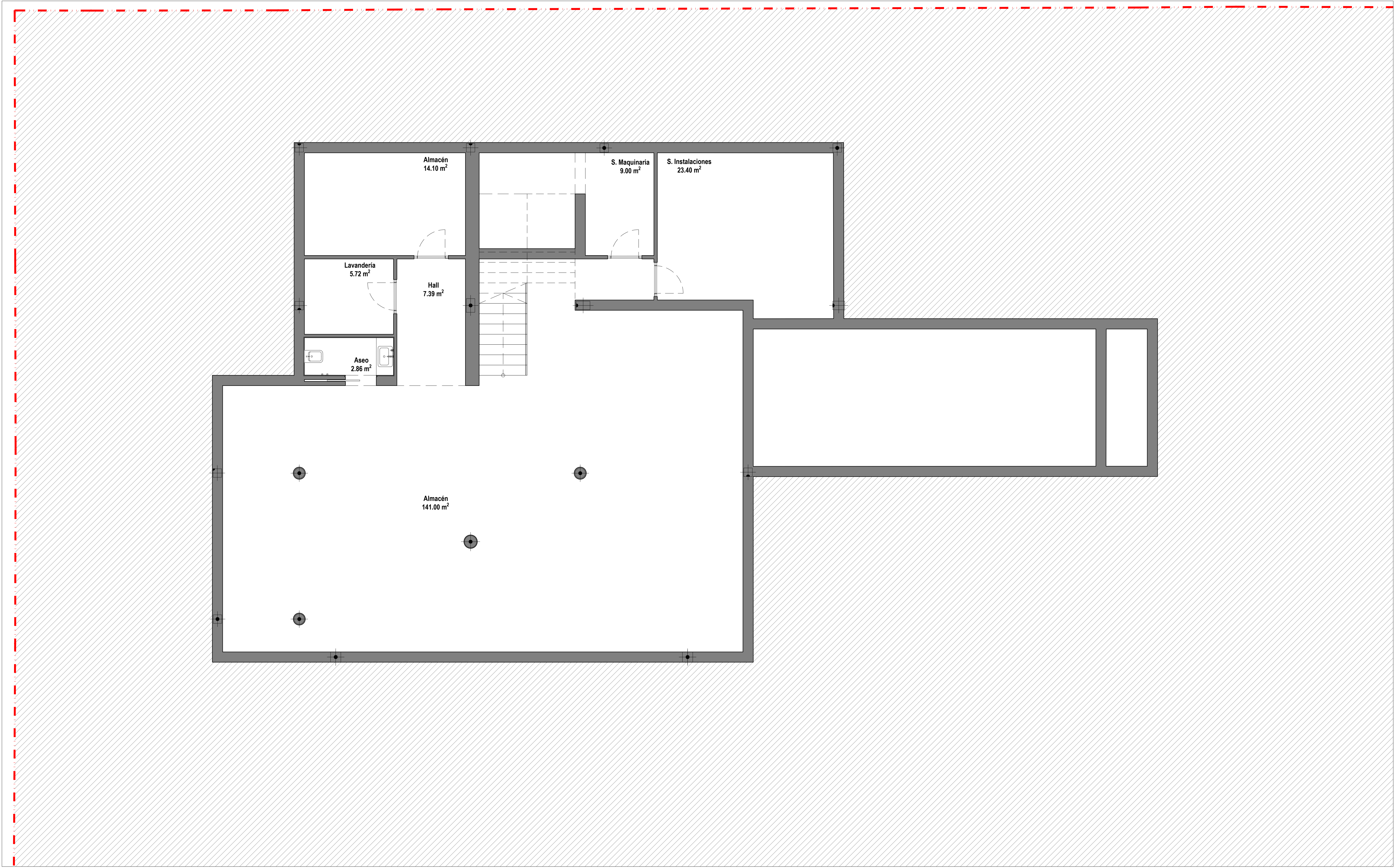
PLANTA SÓTANO_E:1.50
