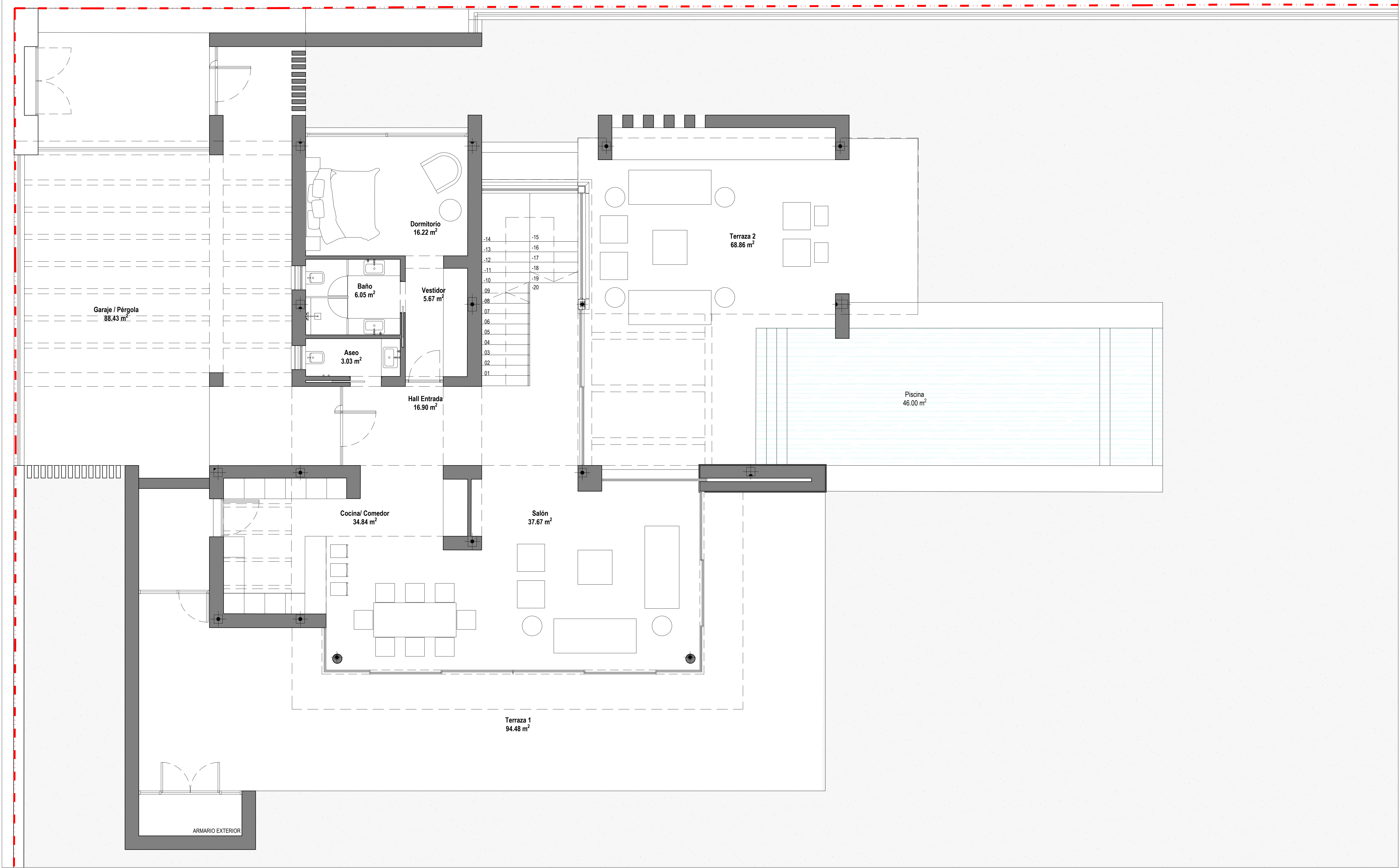
PLANTA BAJA_E:1.50
