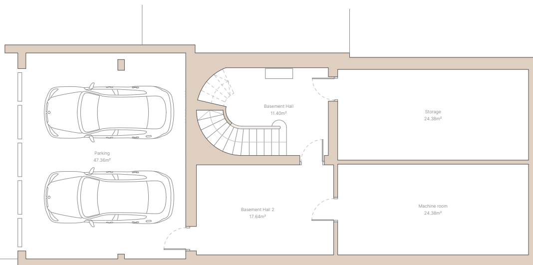
PLANTA SÓTANO BASEMENT
